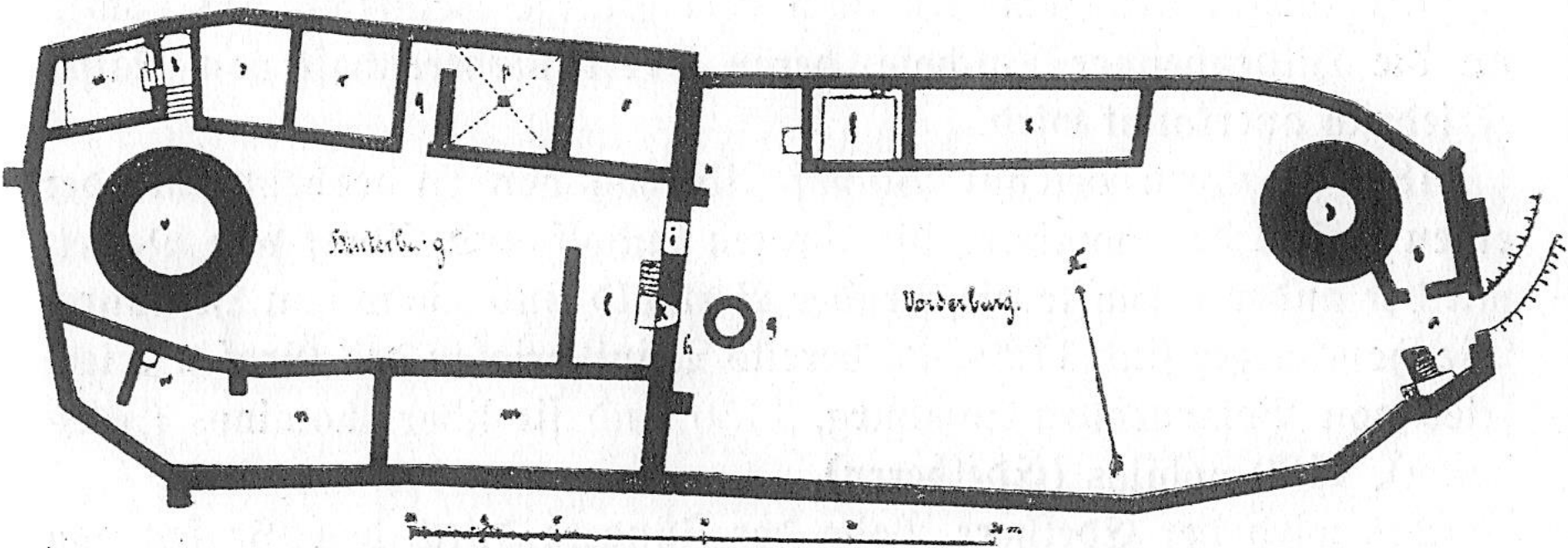
Homburg, Grundriß. (Aus St., B. u. K. D. IV, 184).
