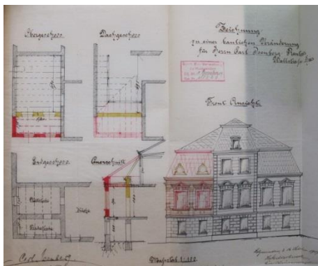
Umbau der Veranda
